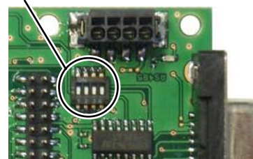
RS-232C/RS-485 切替えスイッチの設定 (左端が#1)
