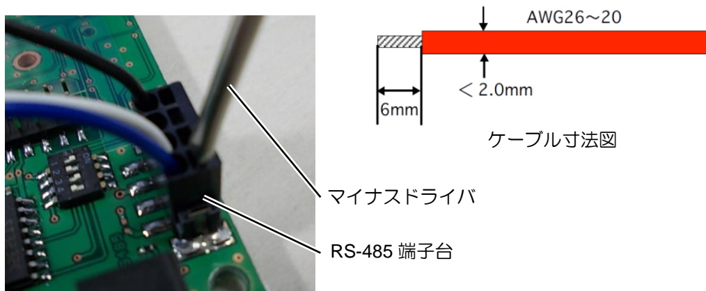
図4 RS-485 端子台へのケーブル配線の様子
