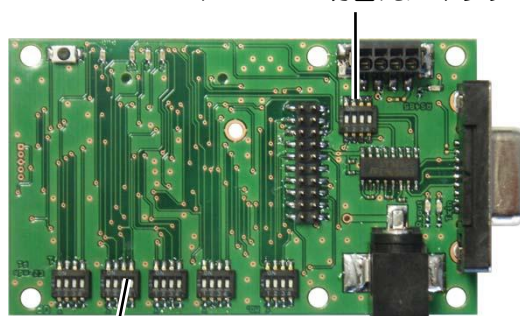
ディップスイッチ SW2
