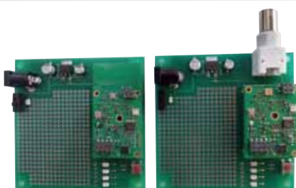
・TS03GRX-EVL 4接点用評価ボード
