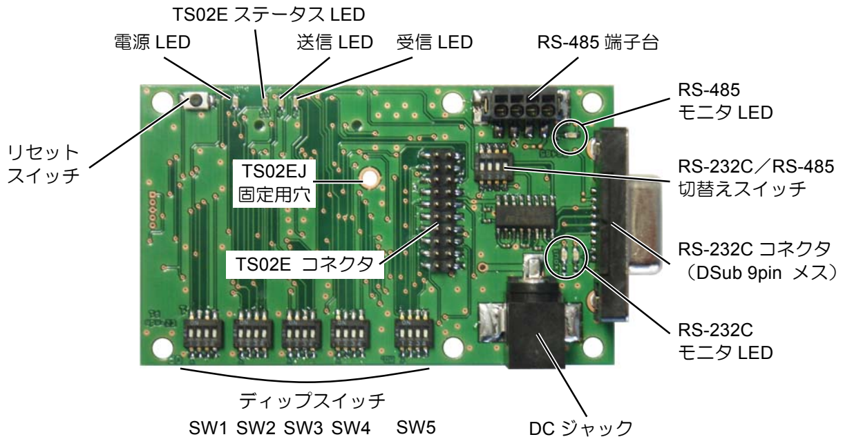
図1 各部の名称
