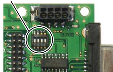
RS-232C/RS-485 切替えスイッチの設定 (左端が#1)
