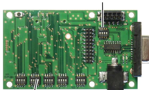
ディップスイッチ SW2
